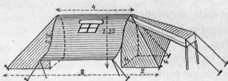
Gibus-tent zonder tenttouwen, voor 16 zieke militairen.
