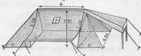
Gibus-tent met rechte bamboes of houten stijlen voor 14 lijders.
