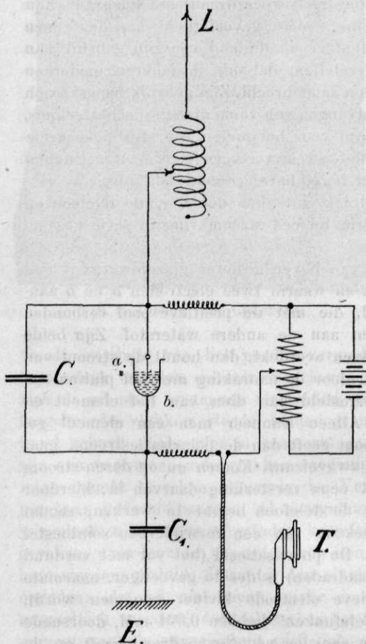
FIG. 10. Electrolytische detector van SCHLOEMILCH. werken van de cel door mid-
