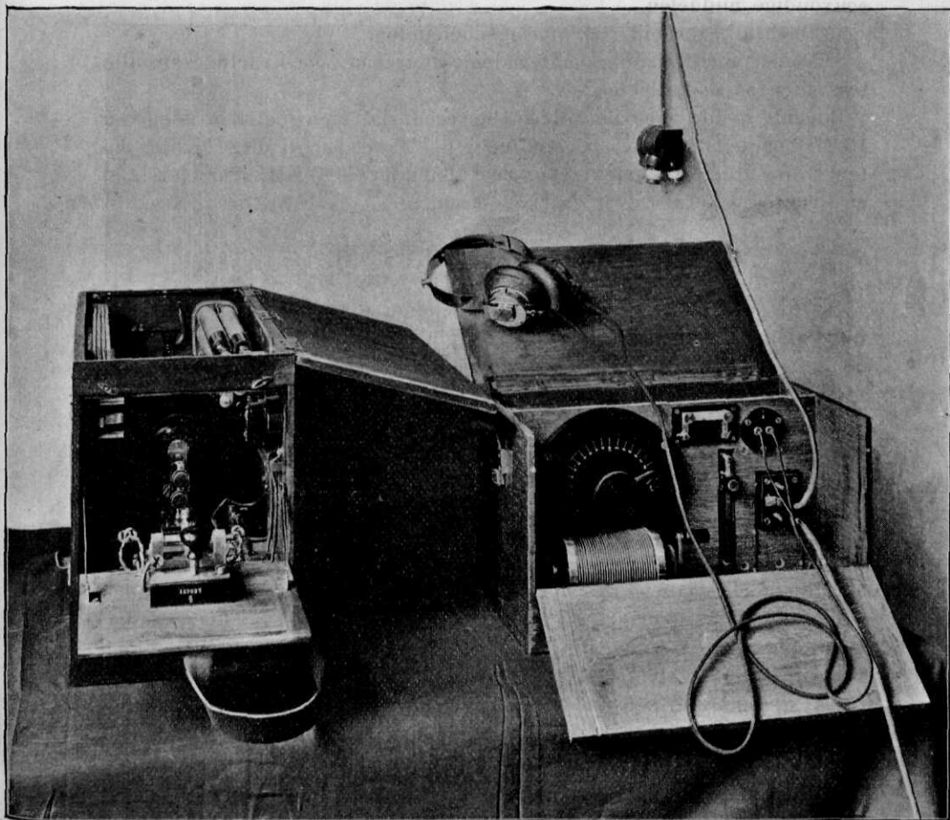
FIG. 11. Draagbaar station voor vonkentelegrafie.
