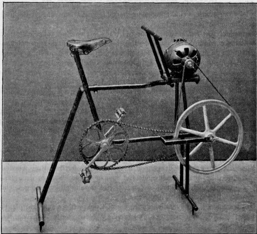
FIG. 12. Trapdynamo voor draagbare stations.
