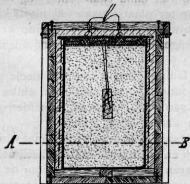
Figuur 16a. Hoogte-doorsnede.
