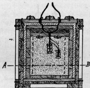
[Figuur 13b. Hoogte-doorsnede. Figuur 13.]
