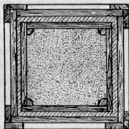
Figuur 13c. Doorsnede A-B op Figuur 13b.
