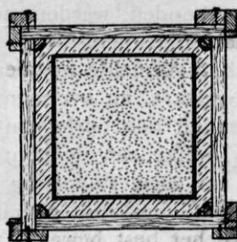
Figuur 16b. Doorsnede A-B op Figuur 16a.
