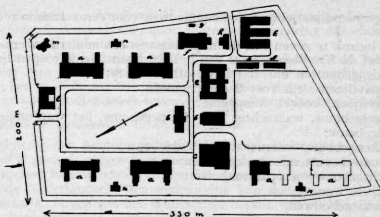
Afb. 7. Kromhoutkazerne te Utrecht . Situatie.
