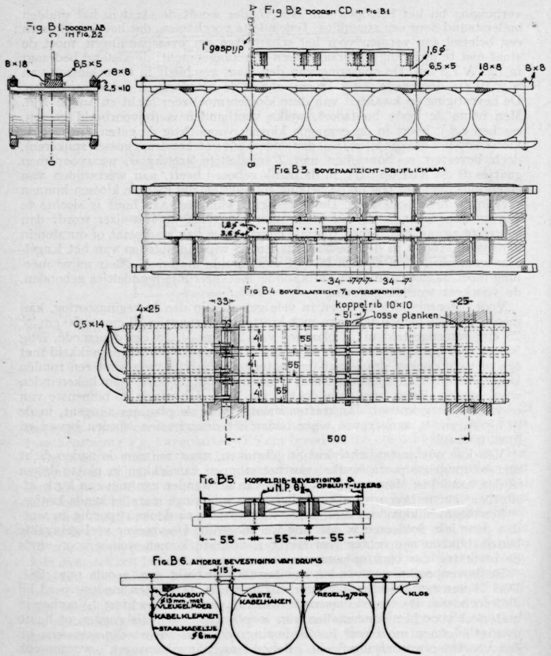
Fig. B. Loopbrug van eenvoudig voorbereid-materieel.
