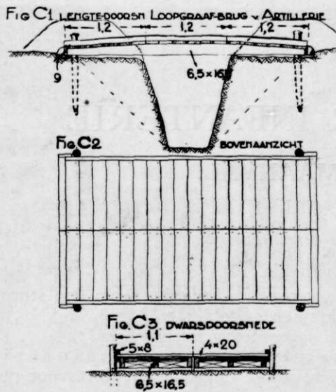
Fig. C. Loopgraafbrug voor veldartillerie. Fig. C 1 . Lengtedoorsnede. C 2 . Bovenaanzicht. C 3 . Dwarsdoorsnede.
