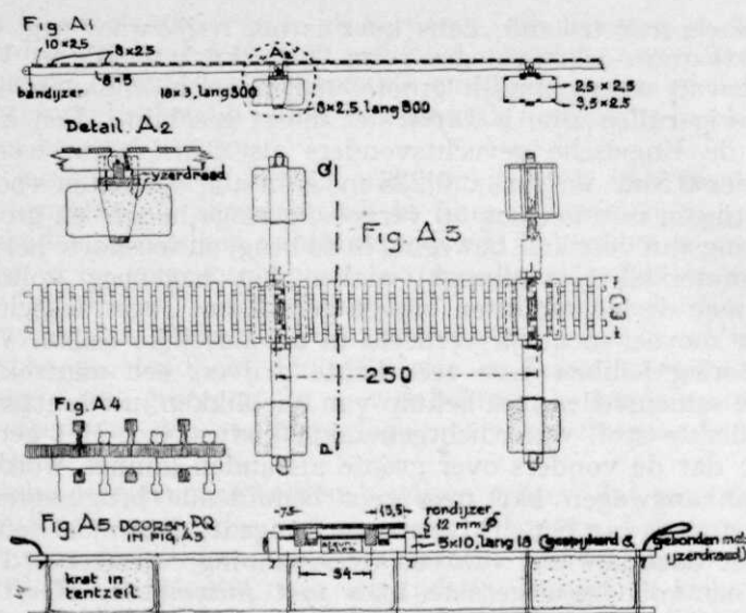
Fig. A. Gevechtsvonder van eenvoudig voorbereid-materieel.
