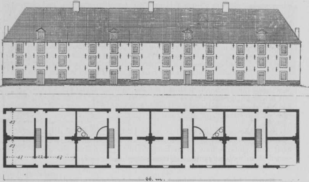
Afb. 3. Kazerne „het Grootte Blok” tē Venlo (1732).
