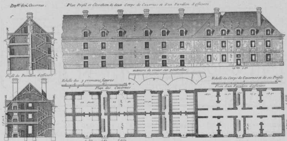
Afb. 2. Inf. kazerne Vauban (einde 17e eeuw).
