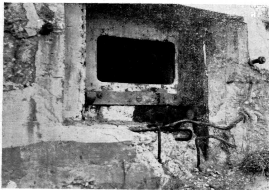
Afb. 7. Voorwand van kazemat 58 S.
