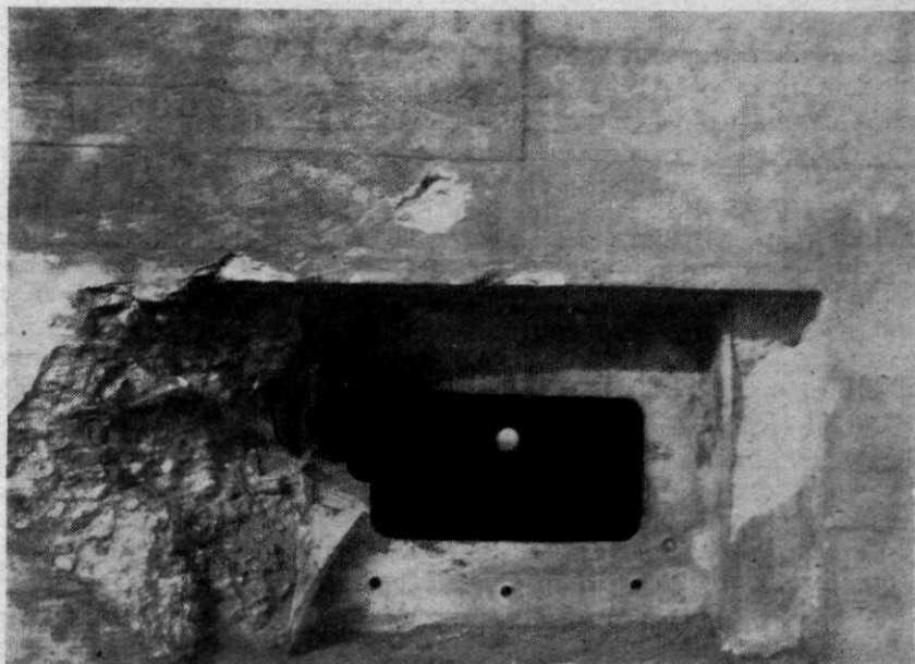
Afb. 12. Kazemat S. 1, frontwand. Treffers door het schietgatraam (links boven).
