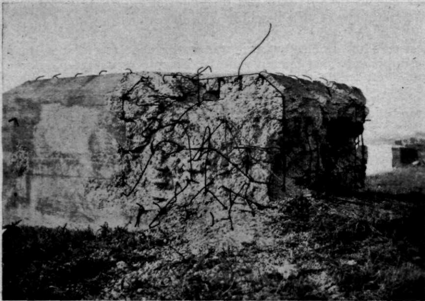
Afb. 6. Kazemat B 5. Flankeerende betonkazemat, aan voorzijde gezien. Zwaar beschadigd door geschutvuur, dat op 2 plaatsen den voorwand doorboorde.
