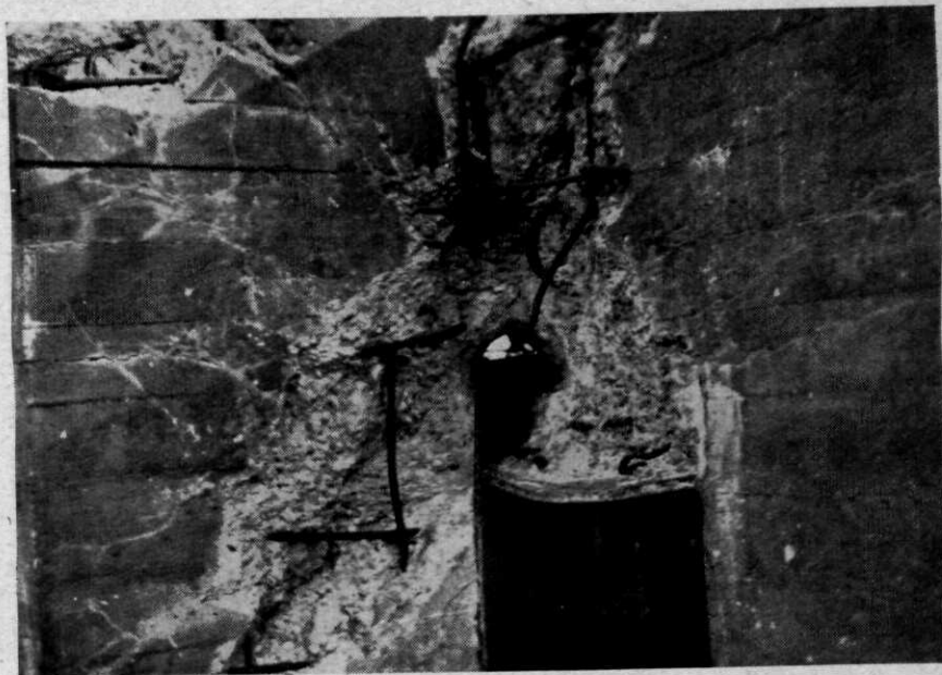
Afb. 7. Kazemat B 5. Gefotografeerd van achteren naar voren. Boven het schietgat een doorboring (doorboorde betondikte 190 cm).
