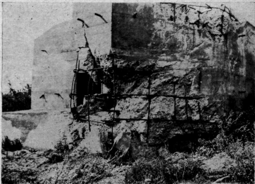
Afb. 11. Kazemat B 2, gezien van de voorzijde. (De kazemat, hoewel als flankerende kazemat ontworpen, schiet frontaal.)
