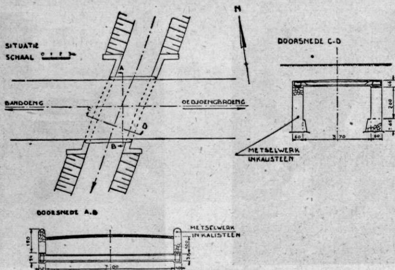
Afb. 12 Gewapend beton aukerplaat op rechtstanden van riviersteen, gebouwd door de 4 genievelddie in de weg Bandoeng—Soemedang
