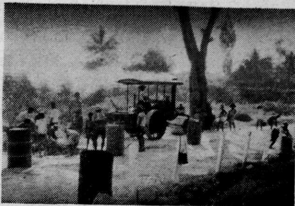
Afb. 8 De slijtlaag wordt ingewalst met weer in bedrijf gestelde oude stoomwalsen
