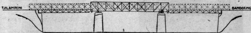
Afb. 19 De nieuwe brug voor gewoon verkeer over de Tji Taroem bij Tjilampeni met gebruikmaking van Bailey als montagebrug volgens ontwerp van de Staatsspoorwegen te Bandoeng
