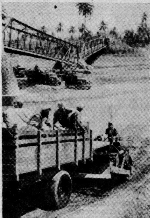
Afb. 14 In de opmars van Tegal naar Pekalongan passeerde de W-brigade de Kali Tjomal door de rivierbedding, hetgeen mogelijk was, doordat een belangrijk deel van het Oost-moessondebiet voor irrigatiedoeleinden was afgetapt
