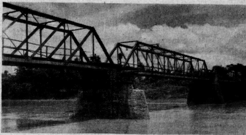
Afb. 15 De Cie legergenietroepen vijzelden de brug over de K. Tjomal onder het verkeer op en herstelden pijler en brugeinden
