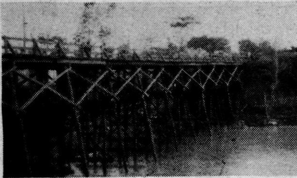
Afb. 10 Houten jukbrug over de Tji Taroem bij Tjilampeni gebouwd door de 16 Cie legergenie troepen. Normaal H.W. komt tot aan de onderzijde van de langschoren
