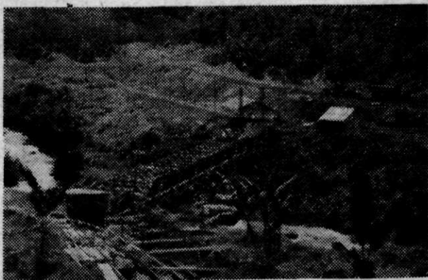
Afb. 7 Vernielde buisleiding van de centrale Djelok ter hoogte van het aquaduct over de K. Toentang. De platgedrukte stalen buis is via de glijd baan van spoorrails op het aquaduct afgevoerd naar de spoorwagens
