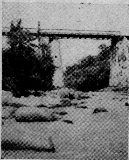
Afb. 5 Baileybrug op 3 steunpunten type 1—1, geslagen door de 6 genievelddie in de weg Tegal—Poerwokerto
