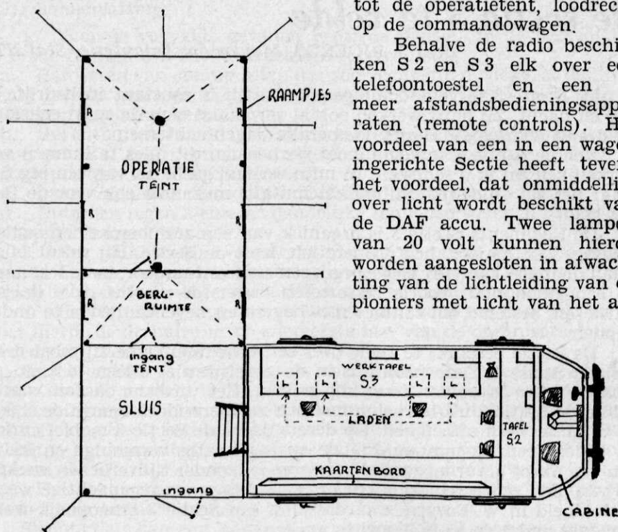
Afb. 1 Opstelling Sectie 3 te velde.
