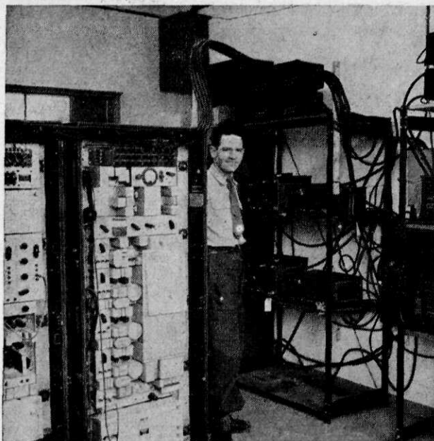
Afb. 7 Opstelling eindapparaat- atuur radiokabels voor vredes-vbdn Staf 1 LK.
