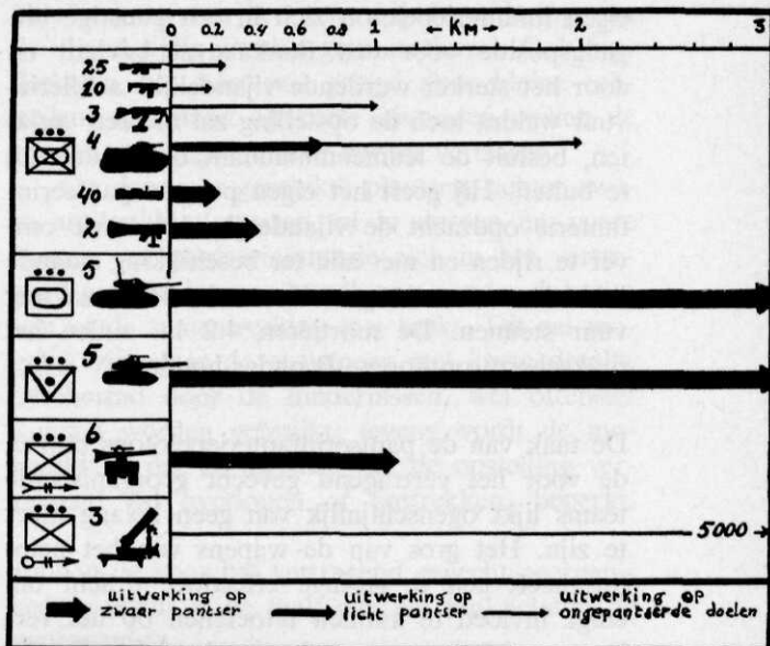
Afb. 3 Schematisch overzicht van de pelotons van de eigen gevechtseenheden met hun voornaamste wapens en de effectieve dracht daarvan
