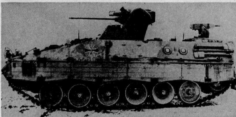
Afb. 13 Marder
