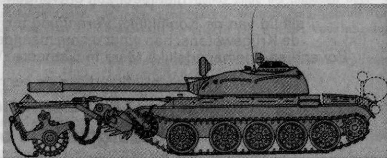
Afb. 3 Combinatie ploeg-roller (KMT-5)
