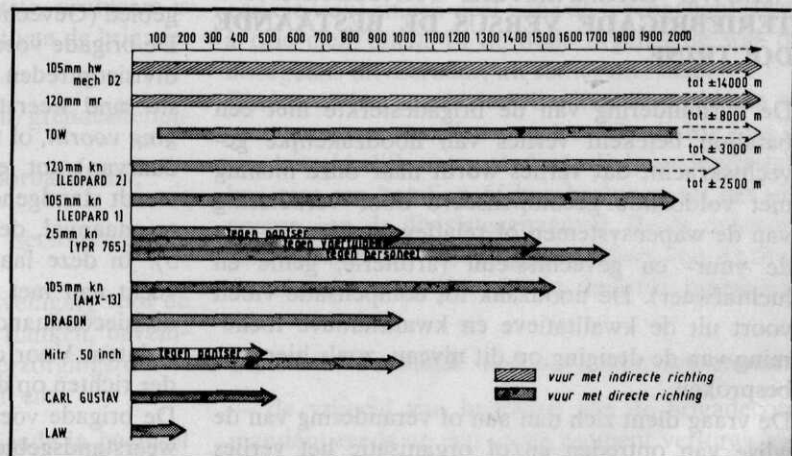
Afb. 4 Effectieve dracht van de belangrijkste wapensystemen, in te zetten uit een steunpunt/grenselstelling
