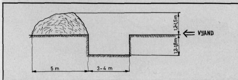
Afb. 5 Rechthoekig profiel
