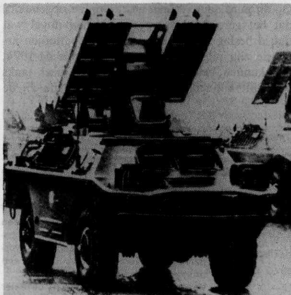
Afb. 3 De Gaskin SA-9; vier lanceerbulzen voor grondluchtraketten gemonteerd op het amfibische BRDM2-onderstel
