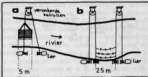
Afb. 5 a. Een eenvoudige constructie voor het vegen van een rivierbodem; b. een speciale constructie voor het vegen van het rivieroppervlak tot een diepte van circa 1,5 m
