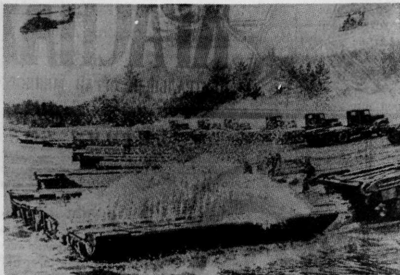
Afb. 10 Het lanceren van de afzonderlijke PMP-pontons; gevechtshelikopters van het type Hind beveiligen de werkzaamheden
