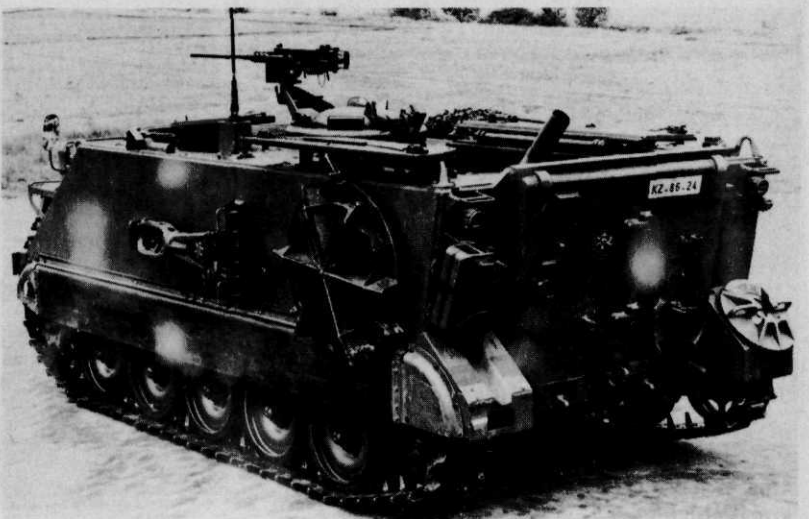
Afb. 8 De 588, Commandovoertuig
