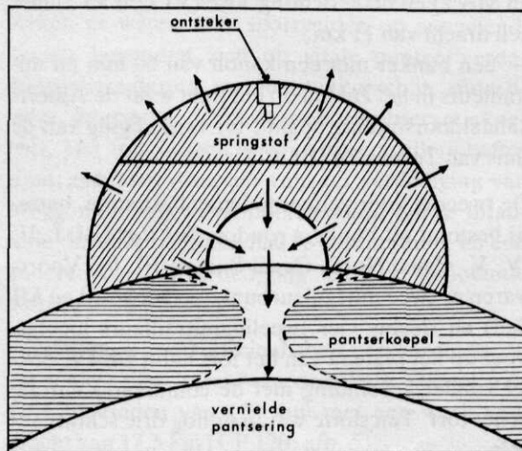
Afb. 8 Tweedelige holle lading van 50 kg (→ geconcentreerde dunne gas- en metaalstraal)
