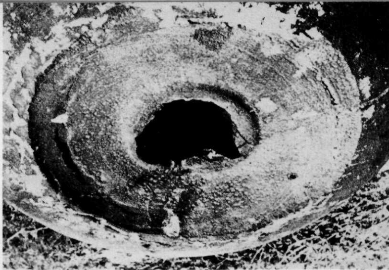
Afb. 9 Uitwerking van de holle lading op een pantserkoepel
