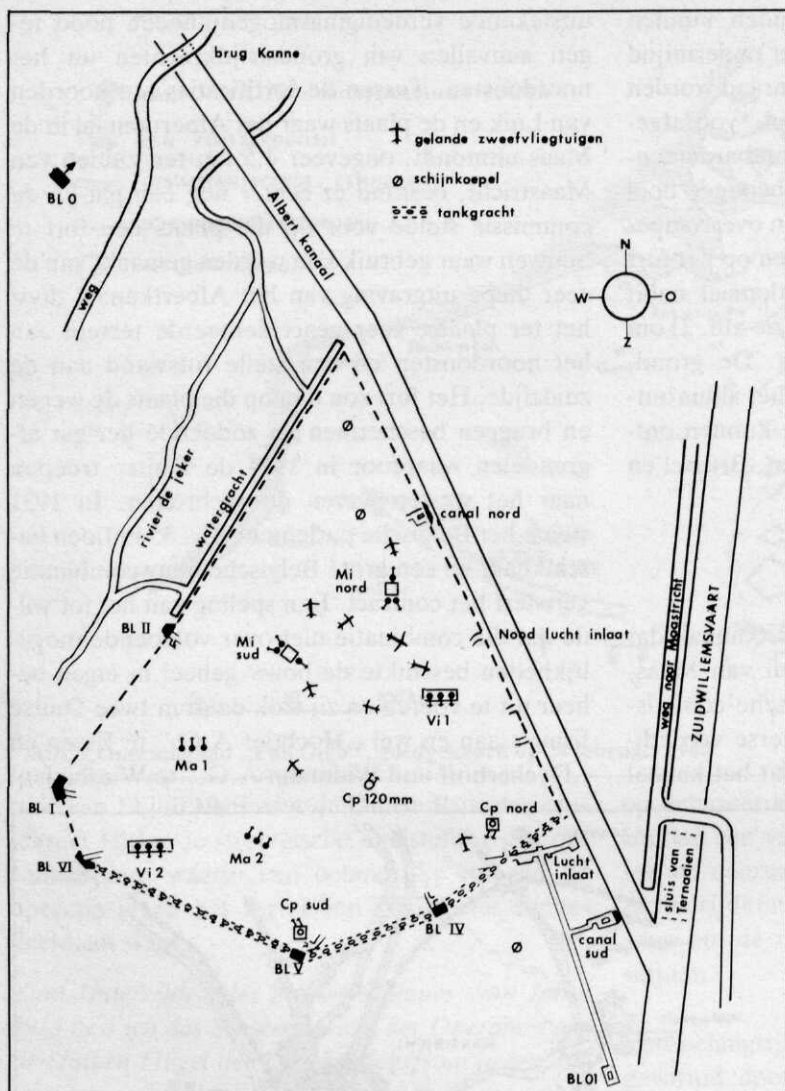
Afb. 3 Installaties fort Eben-Emael
