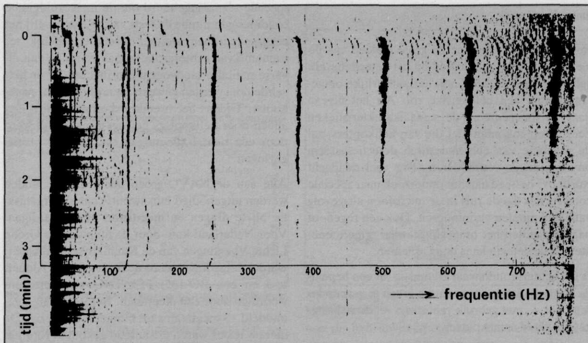
Afb. 8 Lijnspectrum als functie van de tijd van een naderende lichte helikopter; op t = 3 is de afstand ca. 10 km, op t = 0 vliegt de heli over de sensor
