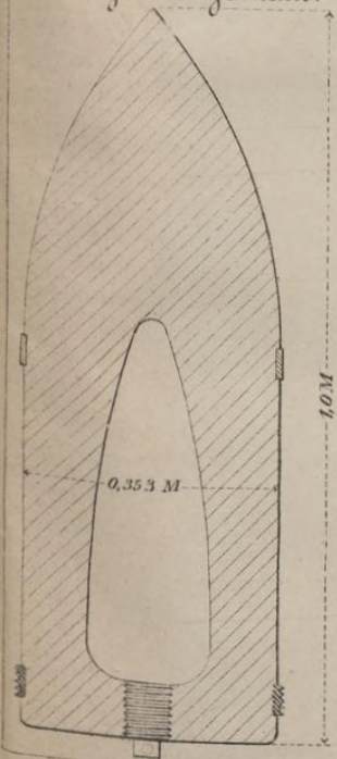
Hardijzeren granaal.
