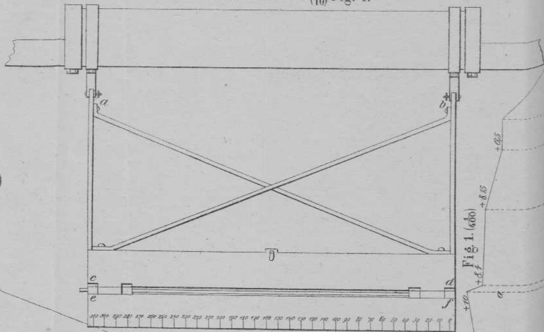
Richtschaal aan het uclijf van achteren (1/10) Fig. 4.
