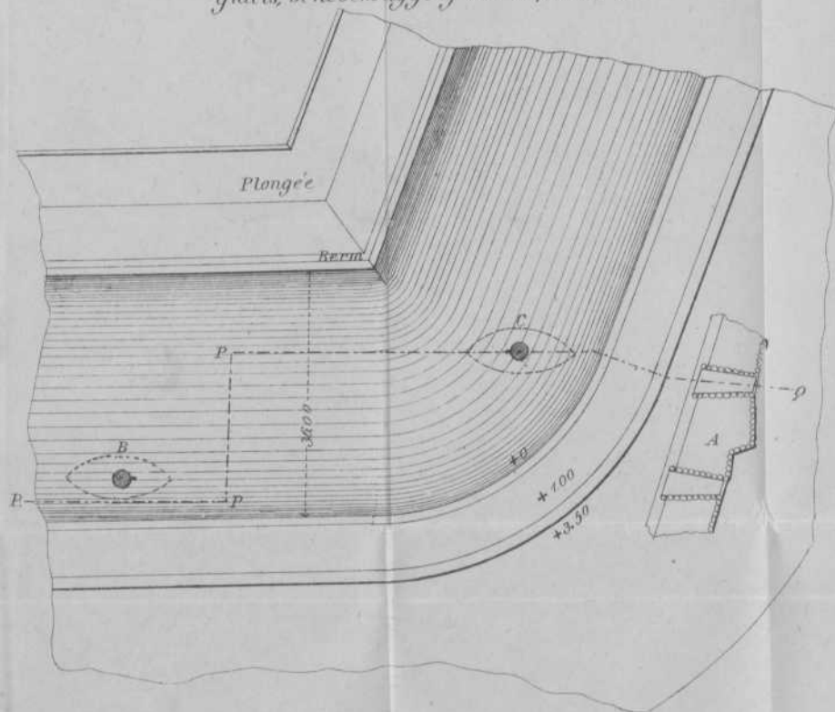
Fig 3. (1000). Platte grond van een fortgracht, met batterij op het glacis, benevens ligging der caponniere.
