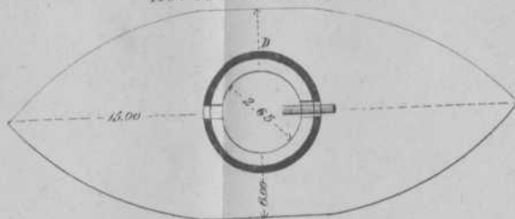
Fig 1. (200). Horizontale doorsnede
