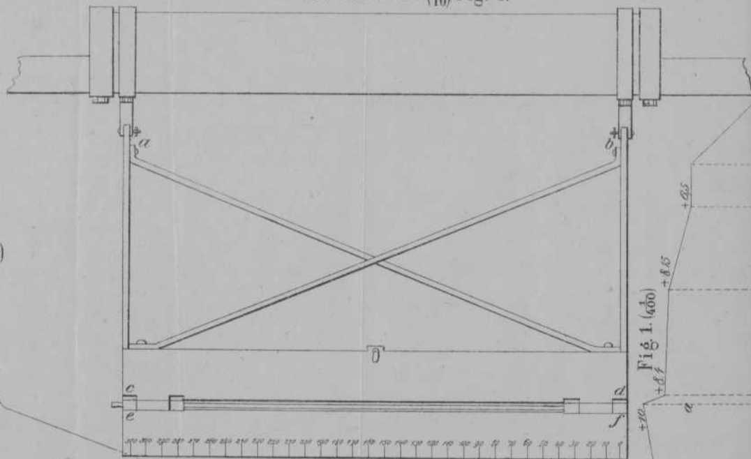
Richtschaal aan het aslijf van achteren ( \frac{1}{10} ) Fig. 4.
