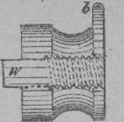
Fig. 4. Opsluitmoer (van onder.)
