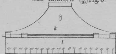
Richtschaal aan den staart van achteren (1/10) Fig. 3.
