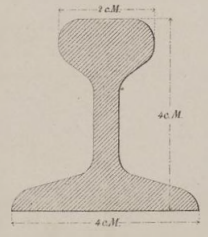
Fig. 1. (1:1) Ijzeren rail van 42 kg per M.
