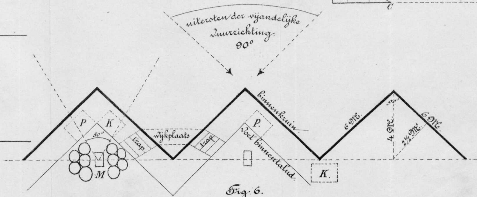
Schets eener mortierbatterij, tegen indirecte, K.F. vuur ontworpen.
