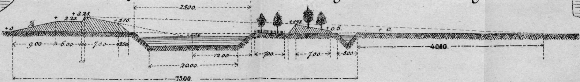
Fig. 3. ( \frac{1}{500} ) Profiel over een bestaanden boogen fortwal met glacis.
