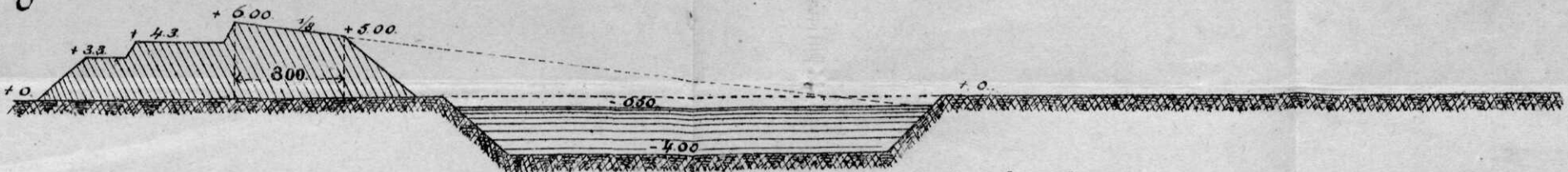
Fig. 6. ( \frac{1}{500} ) Gewijzigd profiel Fig. 5.
