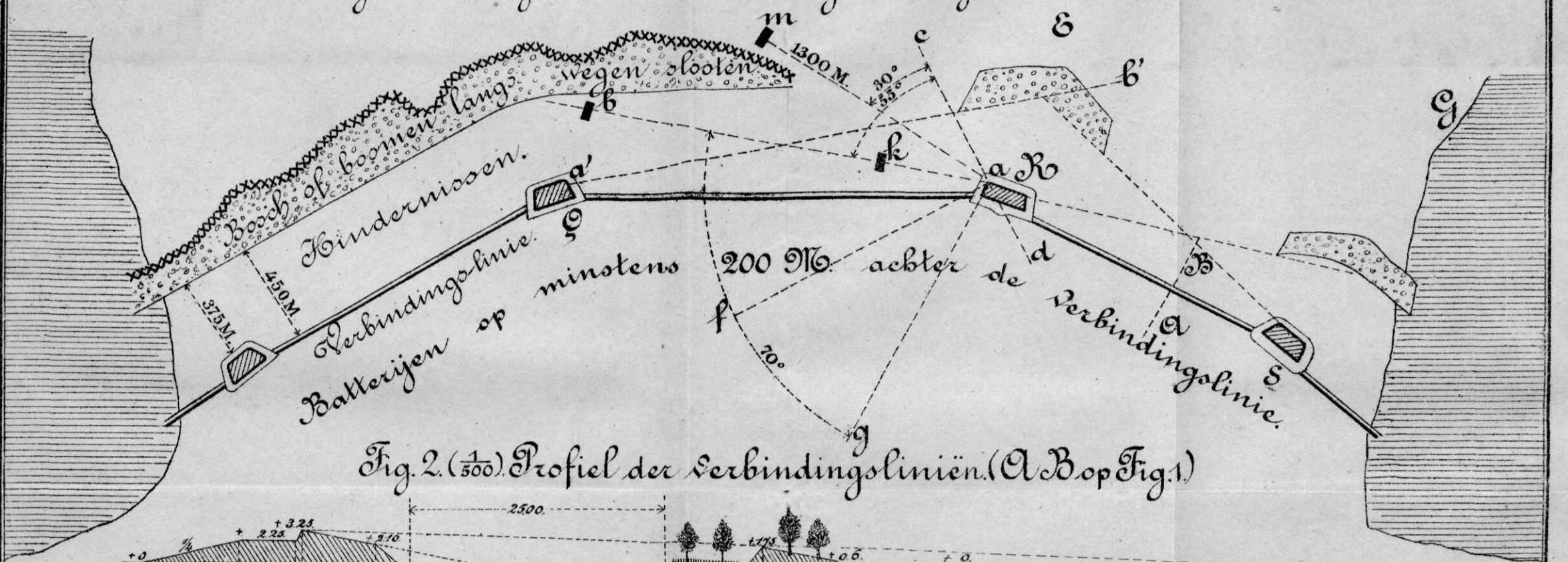
Fig. 1. ( \frac{1}{25000} ) Figuratieve voorstelling van een gedeelte onzer liniën.
