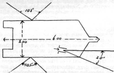
Afb. 1. Schema van de Schneider.
