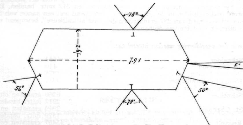
Afb. 2. Schema van de St. Chamond.
